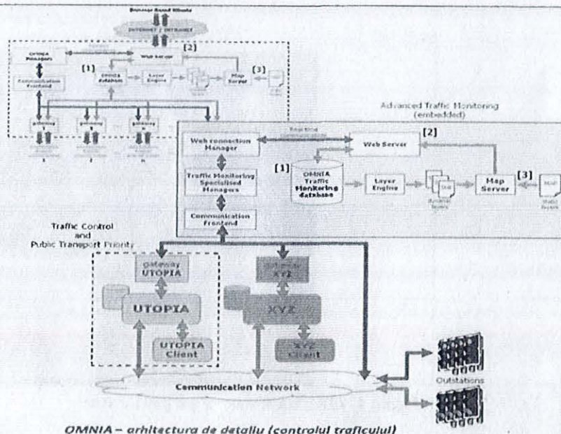
OMNIA - arhitectura de detaliu (controlul traficului)
