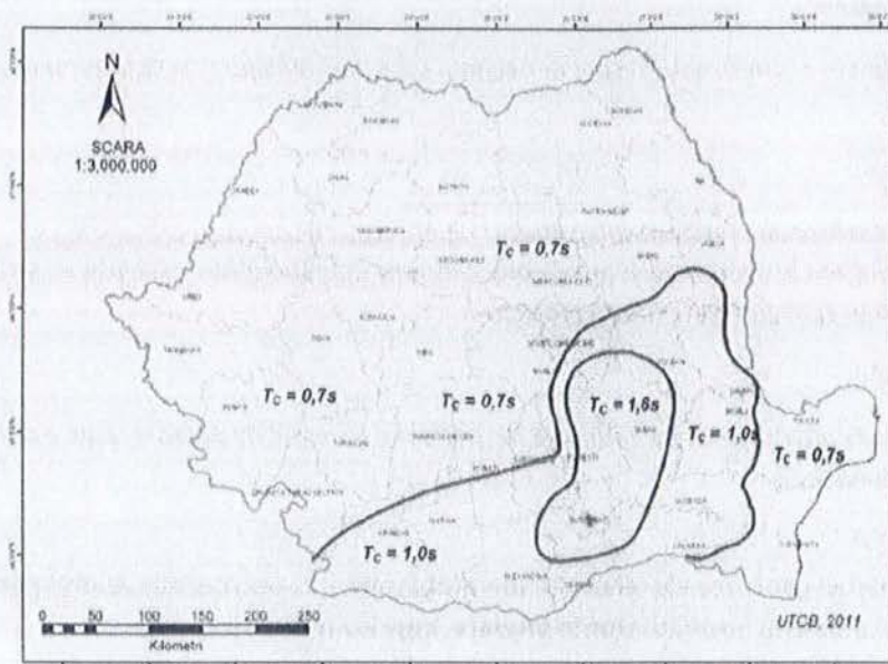
Figura A.2 Zonarea teritoriului României în termeni de perioada de control (colp), T_c a spectrului de răspuns
