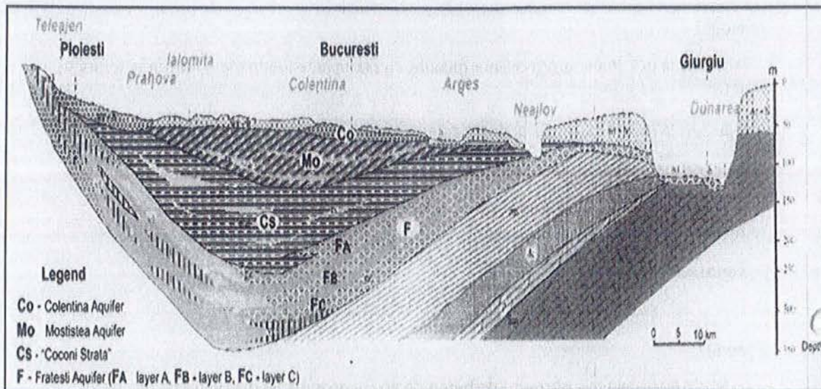
(iv) Fig.3 Sectiune geologica 1 - 1'
